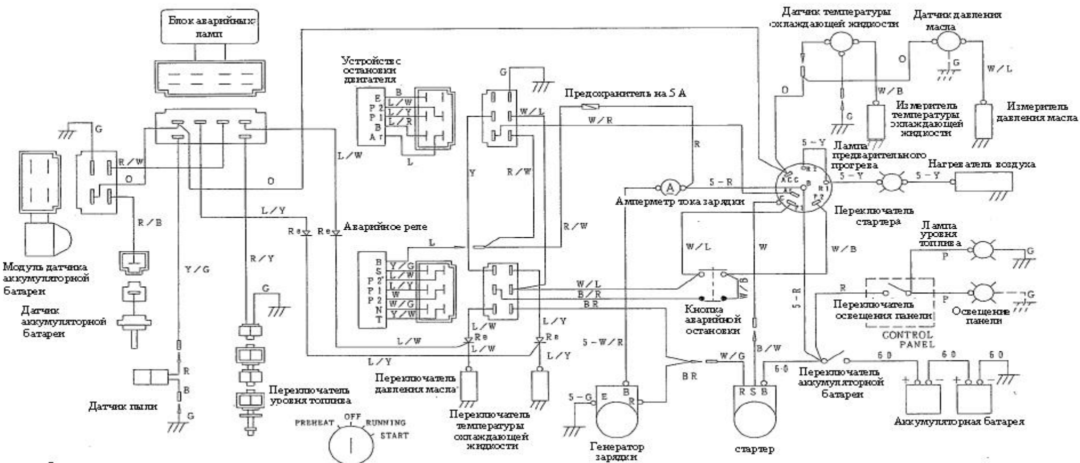
Соединение переключателя стартера
