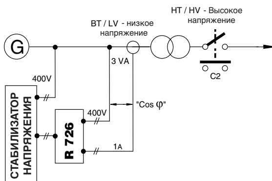
ВСТРОЕННЫЙ СТУПЕНЧАТЫЙ ТРАНСФОРМАТОР - ТОЛЬКО РЕГУЛИРОВКА КОЭФФИЦИЕНТА МОЩНОСТИ
