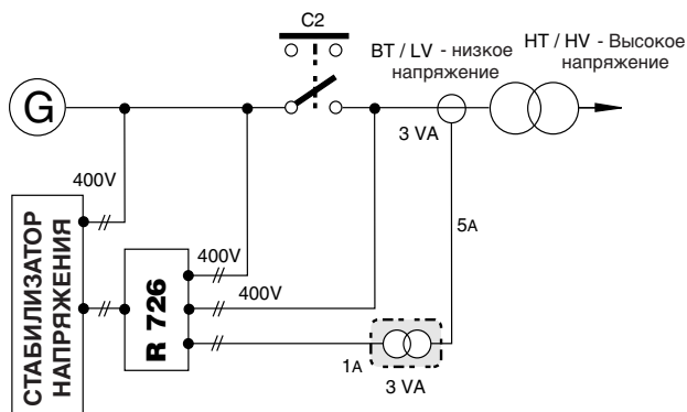
СТАНДАРТНОЕ НИЗКОЕ НАПРЯЖЕНИЕ - ТОК ВТОРИЧНОЙ ОБМОТКИ ТРАНСФОРМАТОРА ТОКА 5 А
